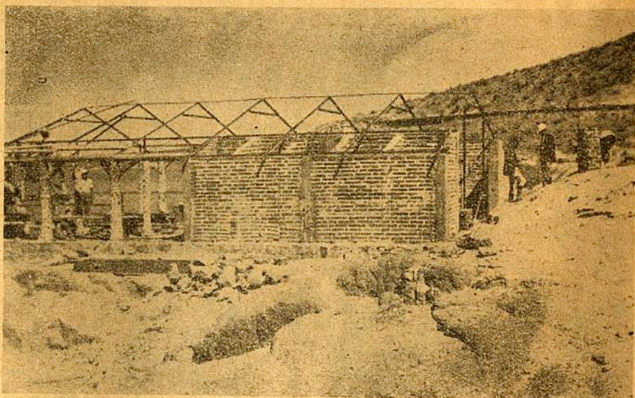
Aspecto de la construcción del Balneario "Coromuel" iniciada el 12 de enero de 1938.
